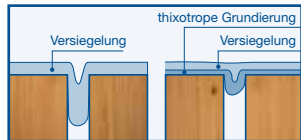
Versiegelung ohne und mit Grundierung
